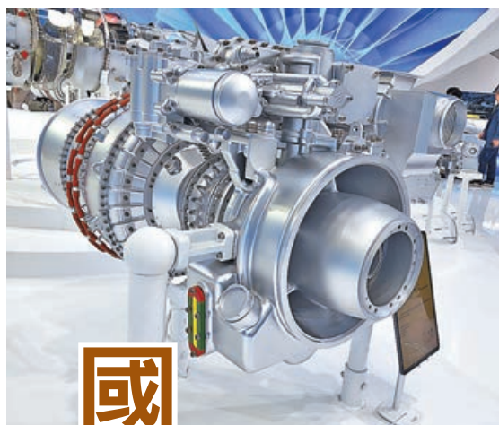
■太行發動機（上圖左）
