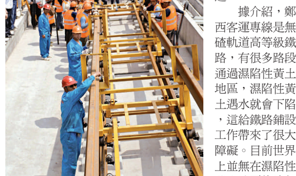
五日，中鐵一局工人開始為鄭西鐵路客運專線陝西段鋪設軌道 (新華社)
