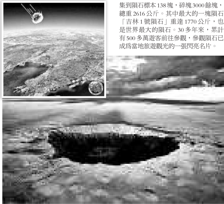
▲美國巴林傑隕石坑是地球上第一個被證實的隕石坑。小圖為地外天體撞擊地球模擬圖 網絡圖片
