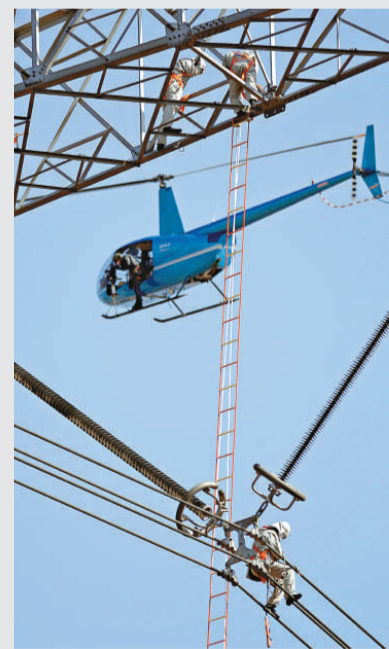
▲十七日，山東省德州平原縣王廟鎮莊村頭，電力作業人員登上56米高的高壓鐵塔，完成了±660千伏電壓等級帶電作業。這是世界上首次在±660千伏高壓線路上進行高空帶電作業 新華社
