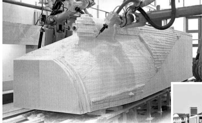
▲「AirMax」船身採用聚亞安酯泡沫材料製造，船體在每次測試前都會清潔乾淨，以最大可能降低表面摩擦力
