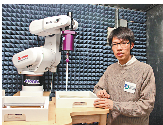
▲陳國雄介紹人體頭部手機輻射量測量儀器
