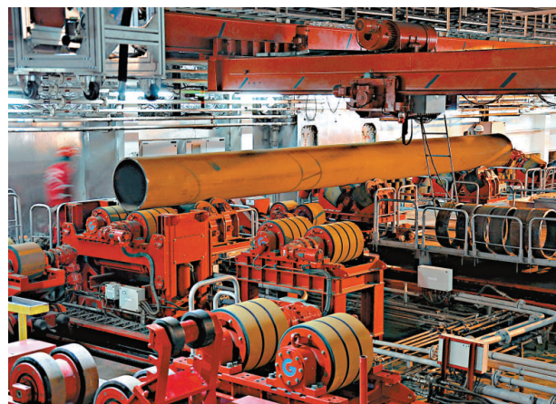
▲38吋鋼管在船艙鋪管機進行加工
