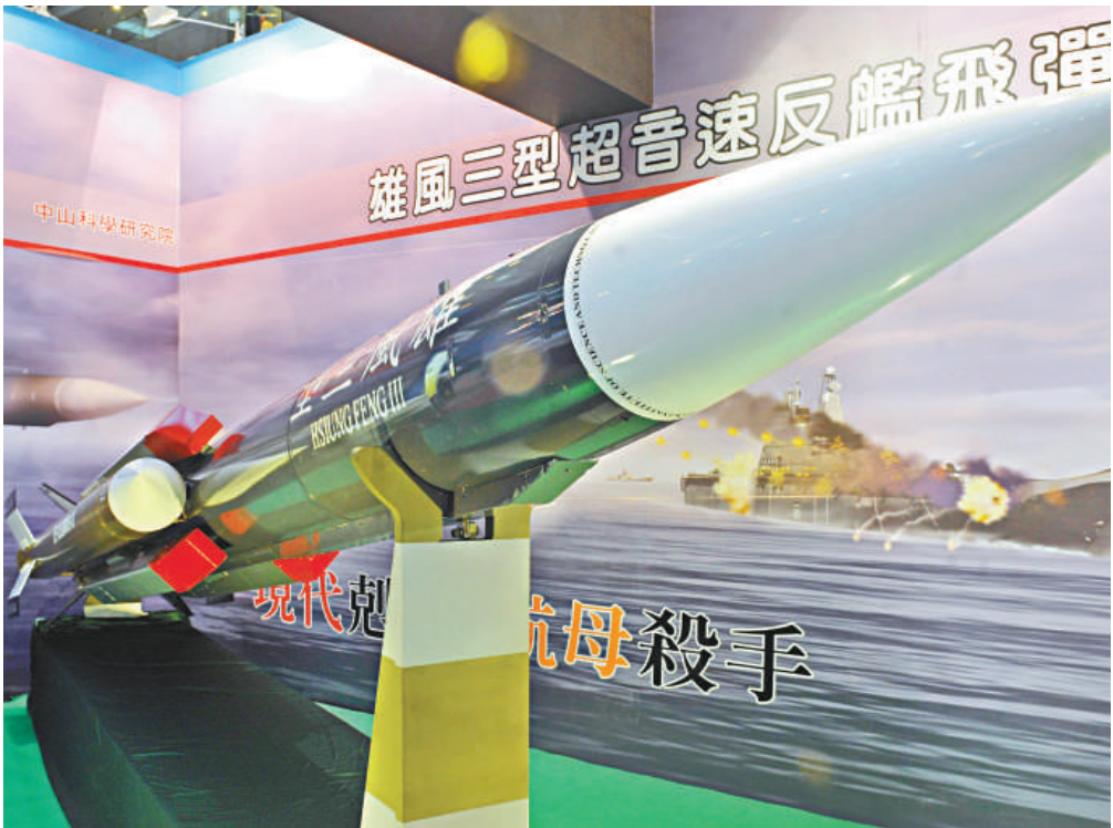
▲長程雄三飛彈傳聞外觀為現役雄三的放大版，圖為現役雄三超音速反艦飛彈 資料圖片
