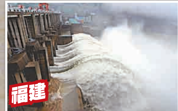
▲5月19日，受庫區上游持續降雨影響，福州水口電站迎來今年入汛以來的首場洪水 新華社
