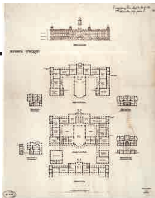
▲一九〇九年十二月香港大學本部大樓的平面圖，翌年大樓動工興建，至一九一二年落成 英國國家檔案館資料
