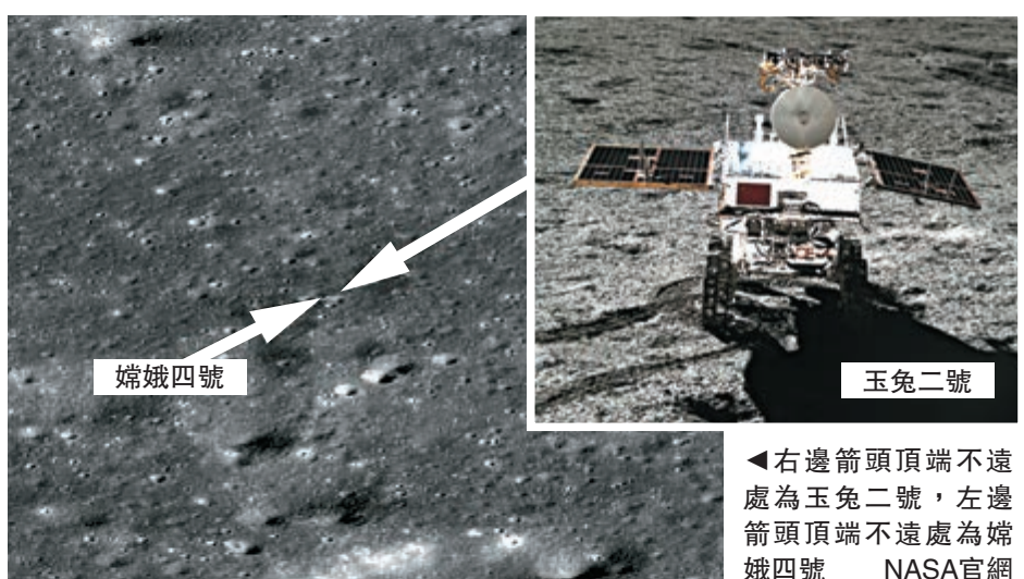
右邊箭頭頂端不遠處為玉兔二號，左邊箭頭頂端不遠處為嫦娥四號 NASA官網
