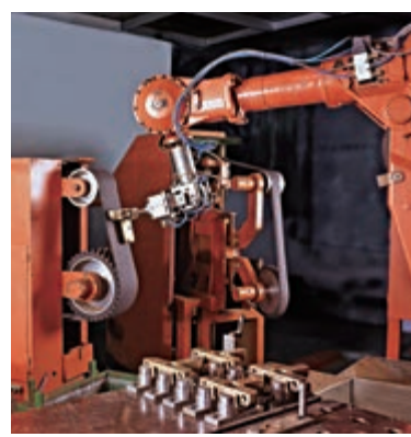
海鷗住工廠房內，機器人正在自動拋磨。受訪者供圖
