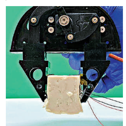
▲楊保博士的團隊將觸覺傳感器安裝在機械手上，能夠成功將豆腐抓住而不捏碎。
