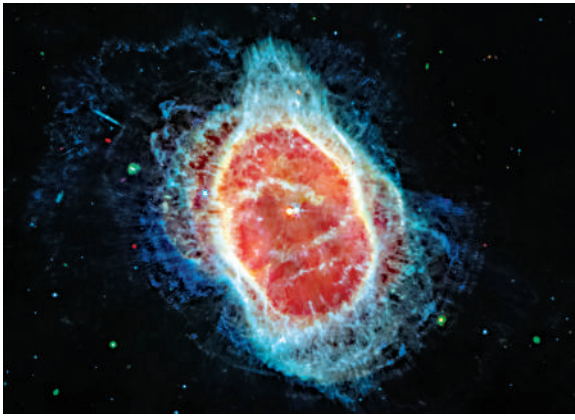
▲中紅外相機拍攝的南環星雲。 法新社
