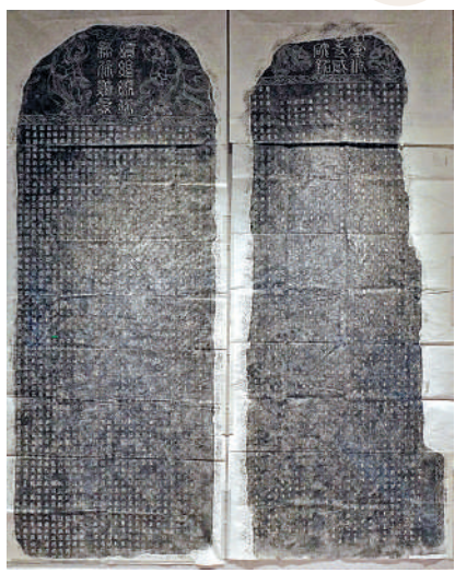
▲西夏碑拓片。
