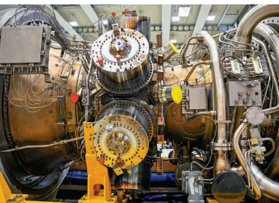
▲「北溪-1」號其中一個渦輪機。法新社
