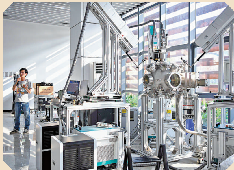
▲工作人員介紹東莞松山湖材料實驗室陳列的超薄膜生產設備。 新華社
