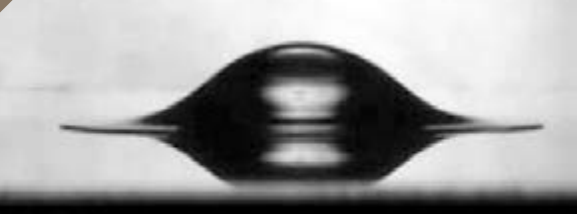
● 近乎真空的低氣壓（17.2kPa）下，水滴在固體表面0.5微秒後的情況。
