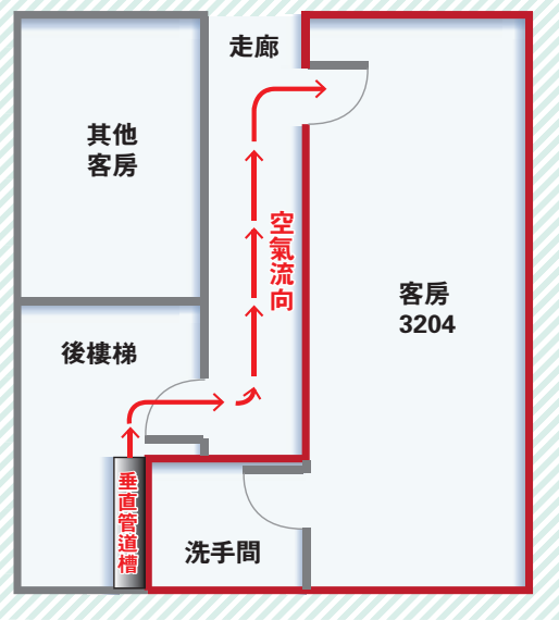
管道槽氣體流入客房示意圖
