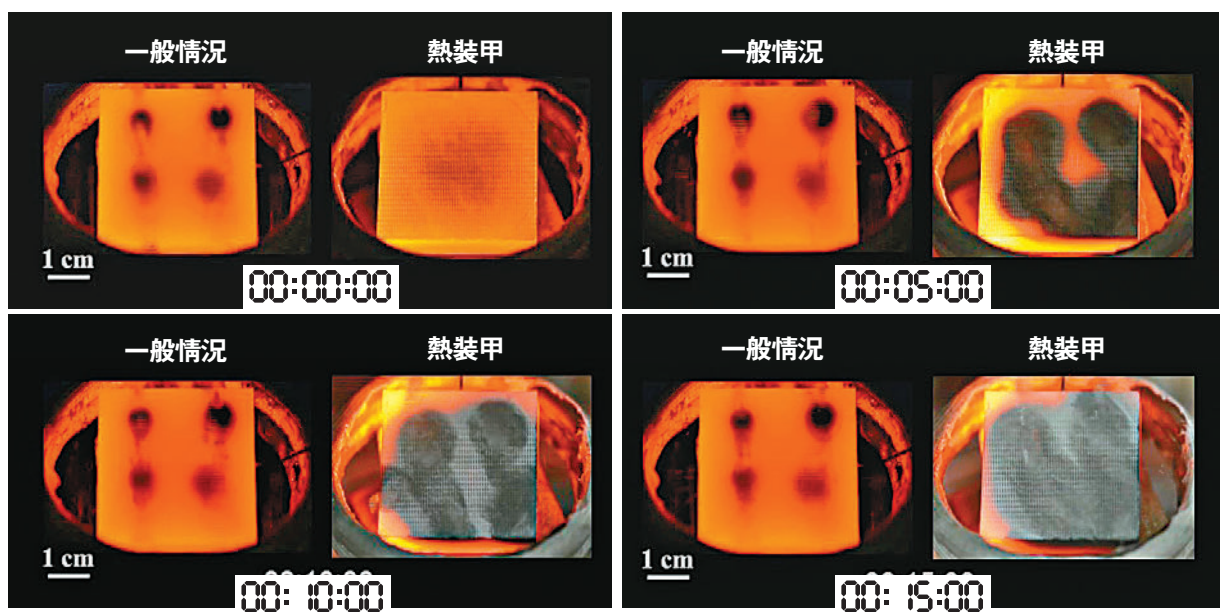
◆研究團隊向1,000℃的超高溫表面持續滴下水滴，受「萊頓弗羅斯特效應」影響，冷卻效能大幅下降；配備熱裝甲後，水滴能快速吸熱蒸發幫助降溫。各圖分別為開始滴水0秒、5秒、10秒及15秒情況。 《自然》片段截圖
