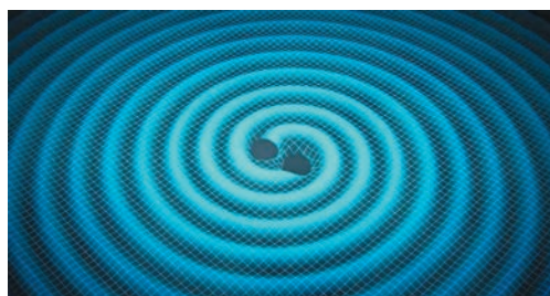
◆重力波成為香港科學家探索暗物質的新利器。 資料圖片
