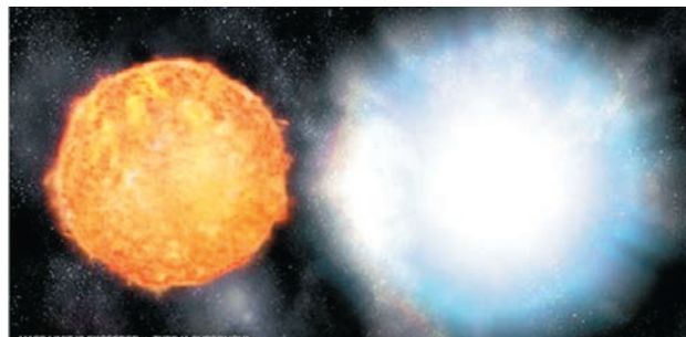
◆白矮星（左圖右方光點）從伴星（左圖左方黃色星球）吸積物質，若白矮星質量增加至超越1.4倍太陽質量，會變得極不穩定，有不受控的核爆反應，成為IA類超新星（右圖）。 NASA圖片
