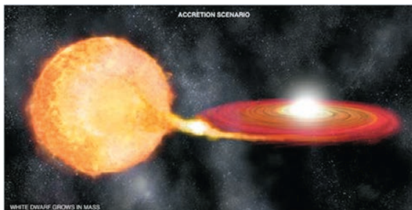
◆白矮星（左圖右方光點）從伴星（左圖左方黃色星球）吸積物質，若白矮星質量增加至超越1.4倍太陽質量，會變得極不穩定，有不受控的核爆反應，成為IA類超新星（右圖）。 NASA圖片
