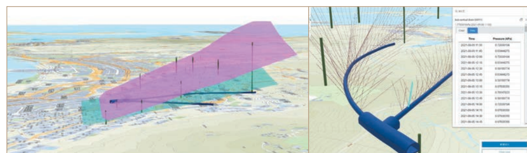
▶運用建築信息模擬技術，將排水隧道、排水斜管、孔隙水壓計，以及周邊環境和地質結構三維圖像化。土力工程處圖片
