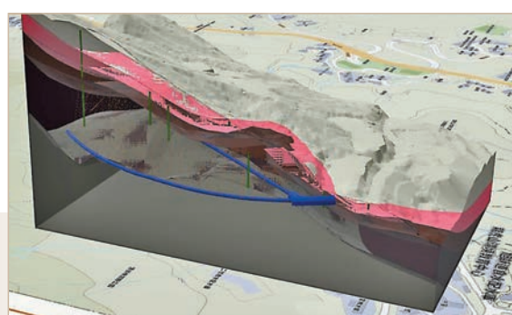
▶運用建築信息模擬技術，將排水隧道、排水斜管、孔隙水壓計，以及周邊環境和地質結構三維圖像化。土力工程處圖片
