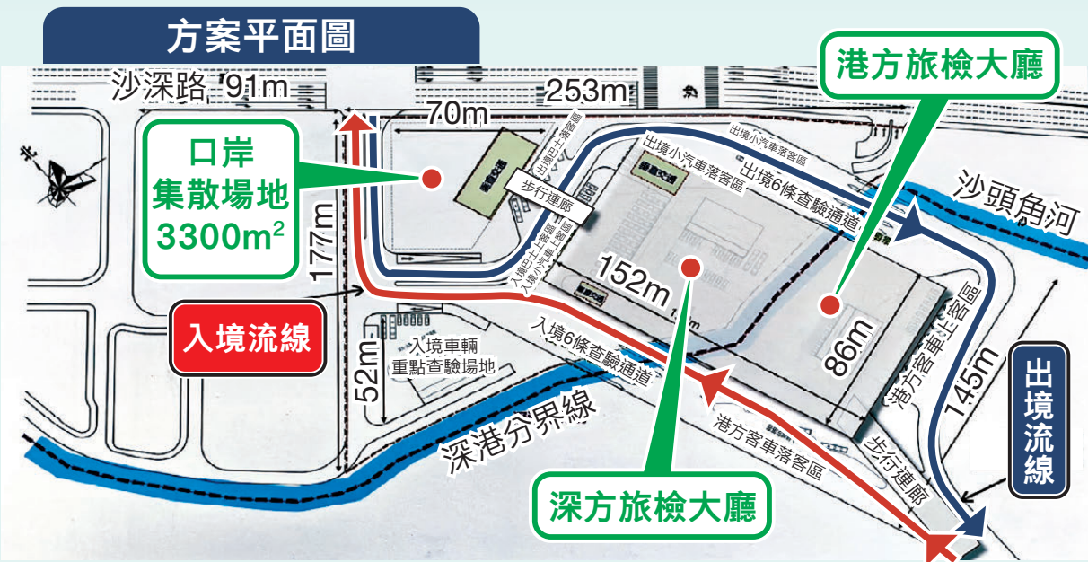
沙頭角口岸重建設計效果圖。香港文匯報深圳傳真
